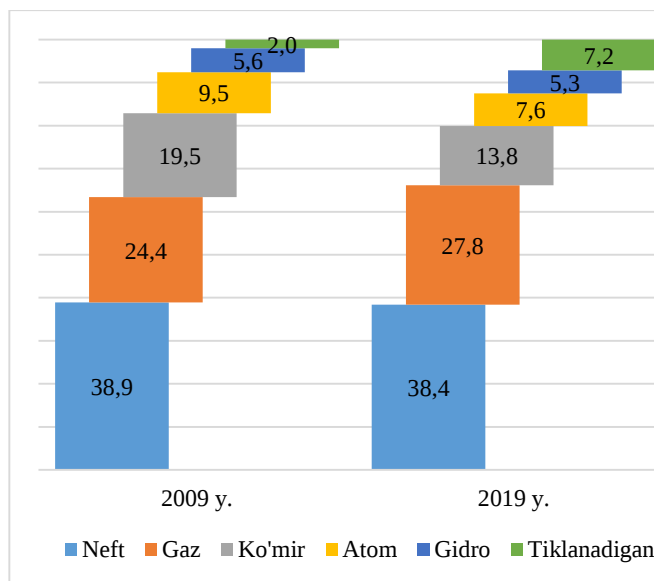
8.1.2-rasm. IHTT mamlakatlarida birlamchi energiya iste'moli tarkibining o'zgarishi, %. 214
