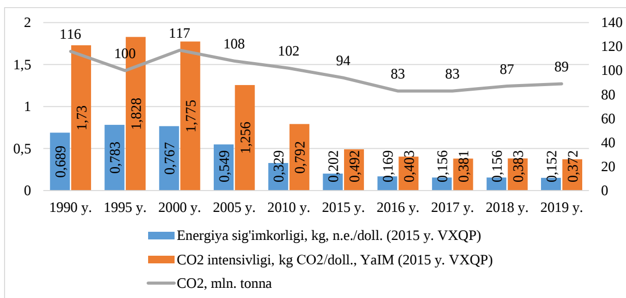
10.2.1-rasm. O'zbekiston iqtisodiyotining energiya samaradorlik ko'rsatkichlari 300
