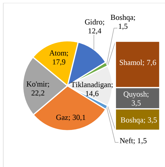
8.1.3-rasm. IHTT mamlakatlarida elektrenergiya ishlab chiqarish manbalari tarkibi, 2019 y. 215
