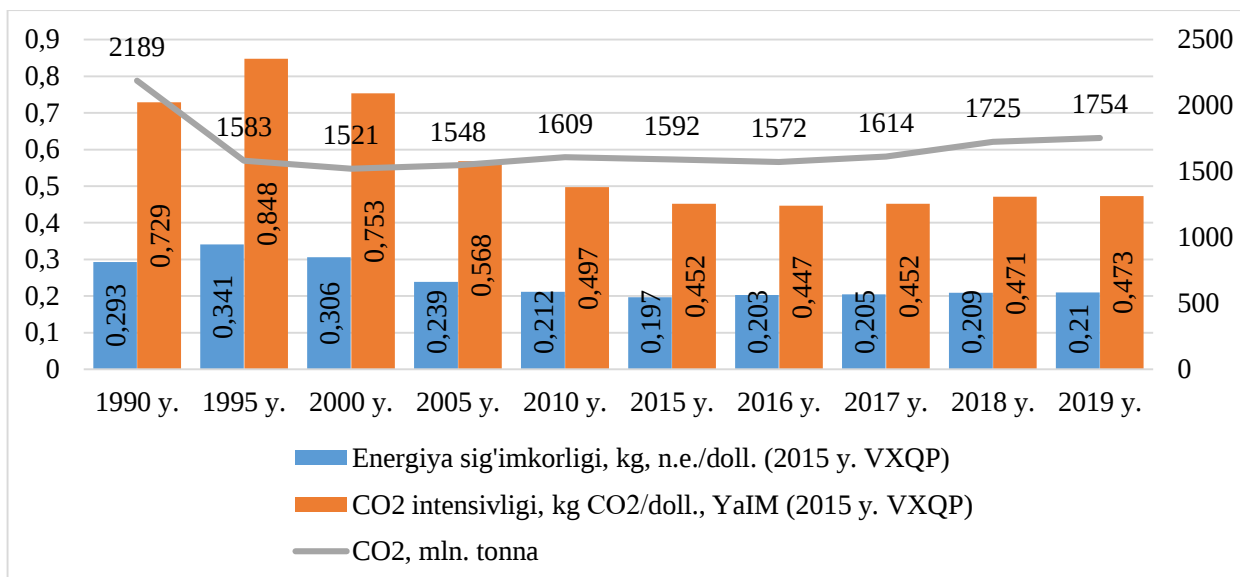
9.3.1.1-rasm. Rossiya iqtisodiyotining energiya samaradorlik ko'rsatkichlari 277
