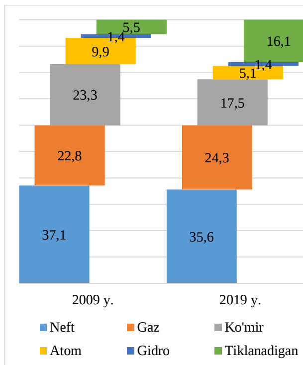
8.4.2-rasm. Germaniyada birlamchi energiya iste'moli tarkibining o'zgarishi, % 245
