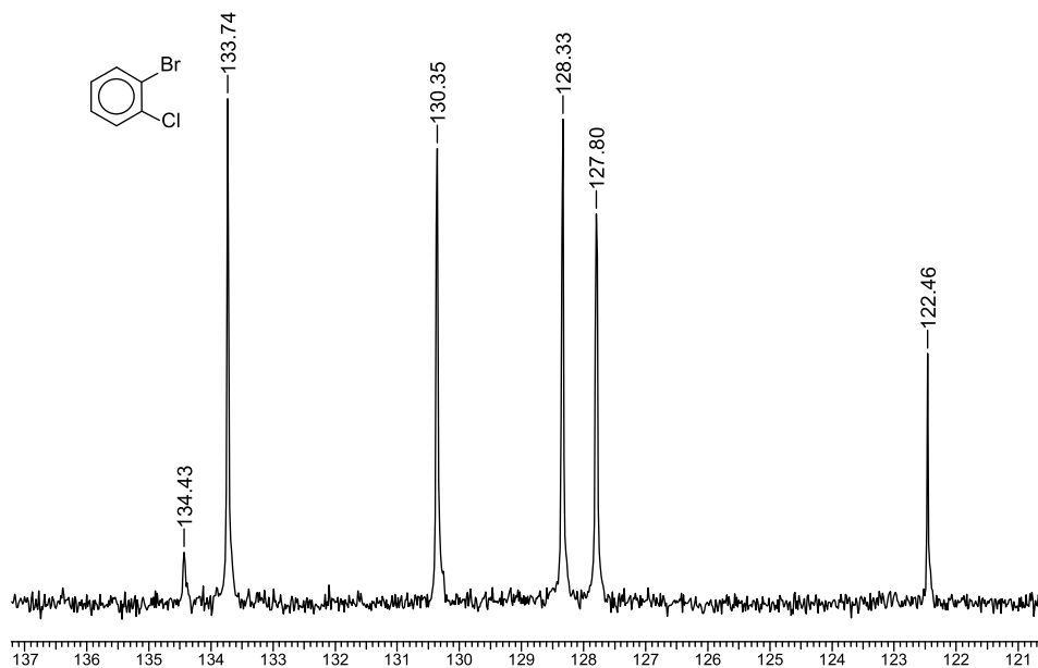
Б10.4. Спектры ЯМР ^1\text{H} и ^{13}\text{C} 2-хлорбромбензола
