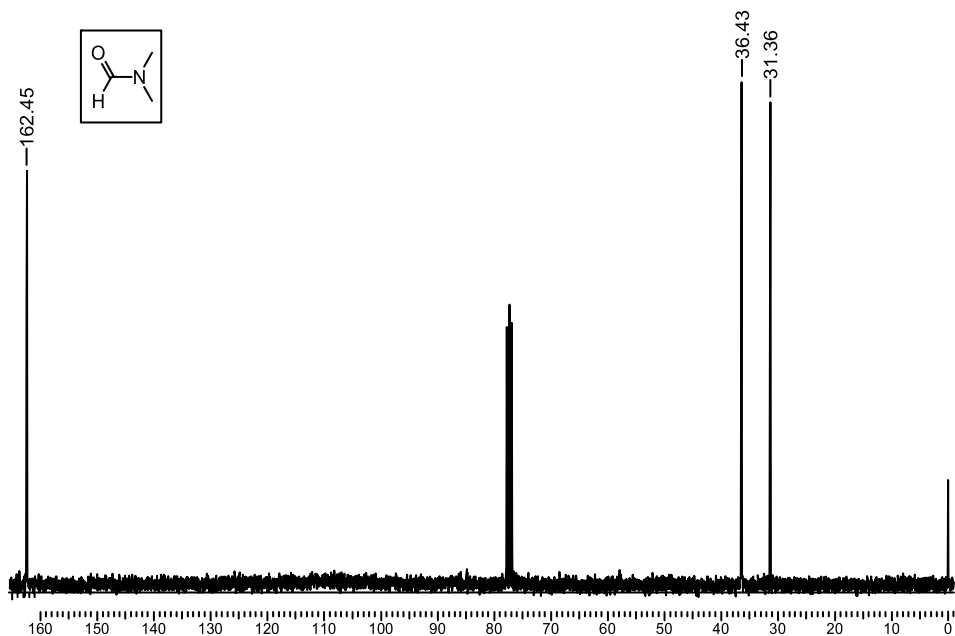
Рис. 88. Спектры ЯМР 1 H и 13 C N,N-диметилформида
