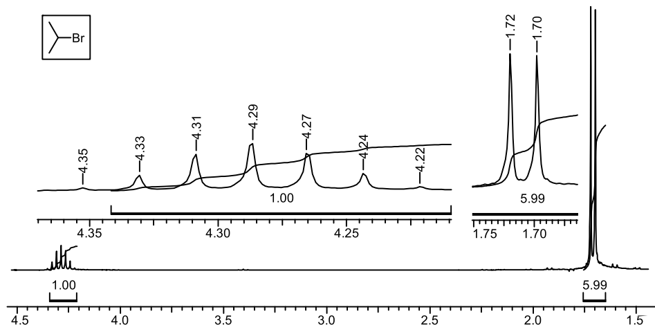
Рис. 65. Пример спиновой системы AX_6 . Сигнал -CH< состоит из 7 спектральных линий. ^3J = [(4.35 - 4.22)/12 + (1.72 - 1.70)/2] \times 300 = 0.0208 \times 300 = 6.25 Гц. КССВ в рутинных спектрах обычно округляют до первого знака после запятой: ^3J = 6.3 Гц
