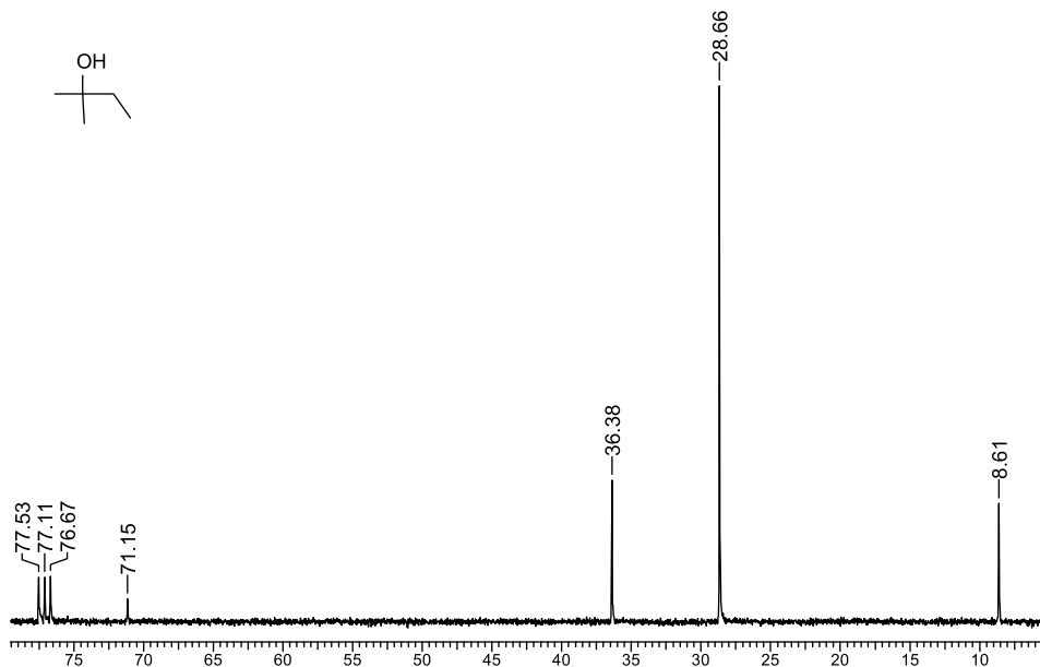
В6.6. Спектры ЯМР ^1\text{H} и ^{13}\text{C} 2-метилбутанола-2
