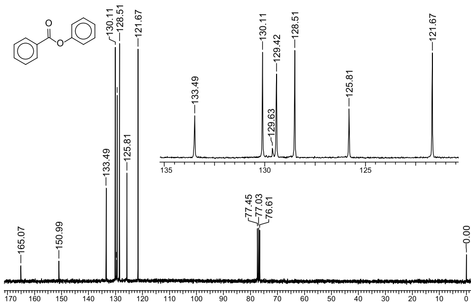
Б1.1.7. Спектры ЯМР ^1\text{H} и ^{13}\text{C} фенолбензоата
