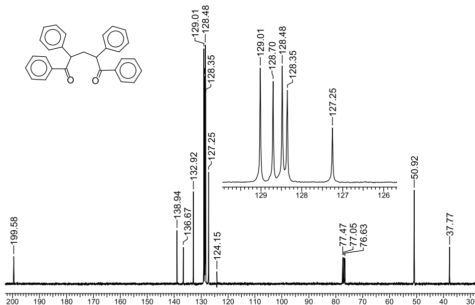
Б4.3.9. Спектры ЯМР ^1\text{H} и ^{13}\text{C} 1,2,4,5-тетрафенилпентандиона-1,5
