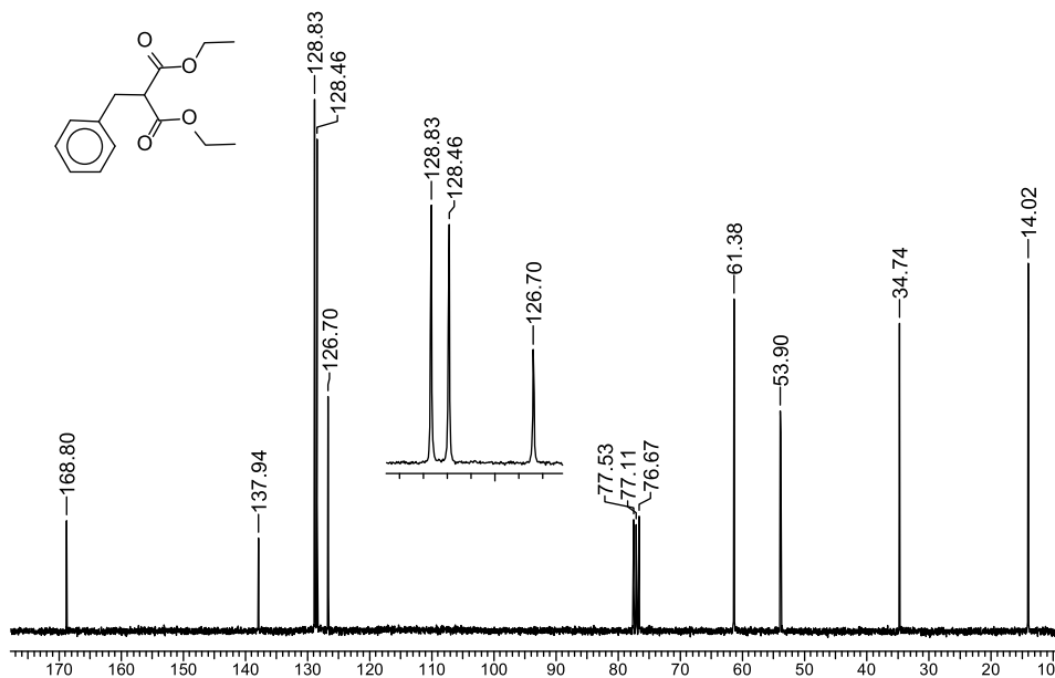
Б5.3.1. Спектры ЯМР ^1\text{H} и ^{13}\text{C} диэтил-2-бензилмалоната
