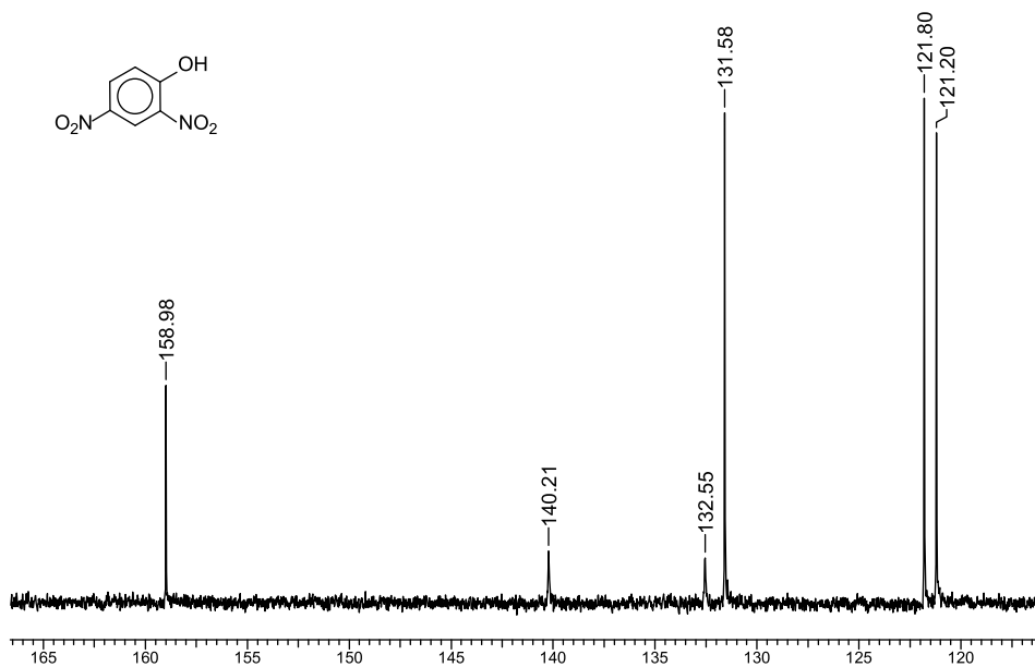
Б8.3. Спектры ЯМР ^1\text{H} и ^{13}\text{C} 2,4-динитрофенола
