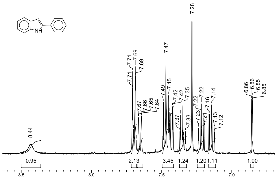
Б11.3. Спектр ЯМР ^1\text{H} 2-фенилиндол.
