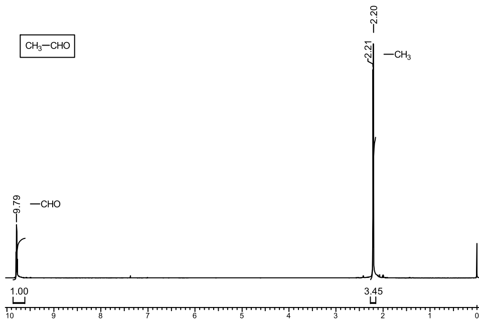
Рис. 52. Спектр ЯМР ^1H ацетальдегида
