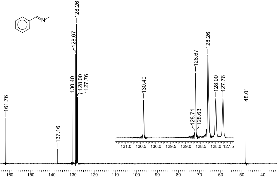
Б4.2.7. Спектры ЯМР ^1\text{H} и ^{13}\text{C} фенилметанимина
