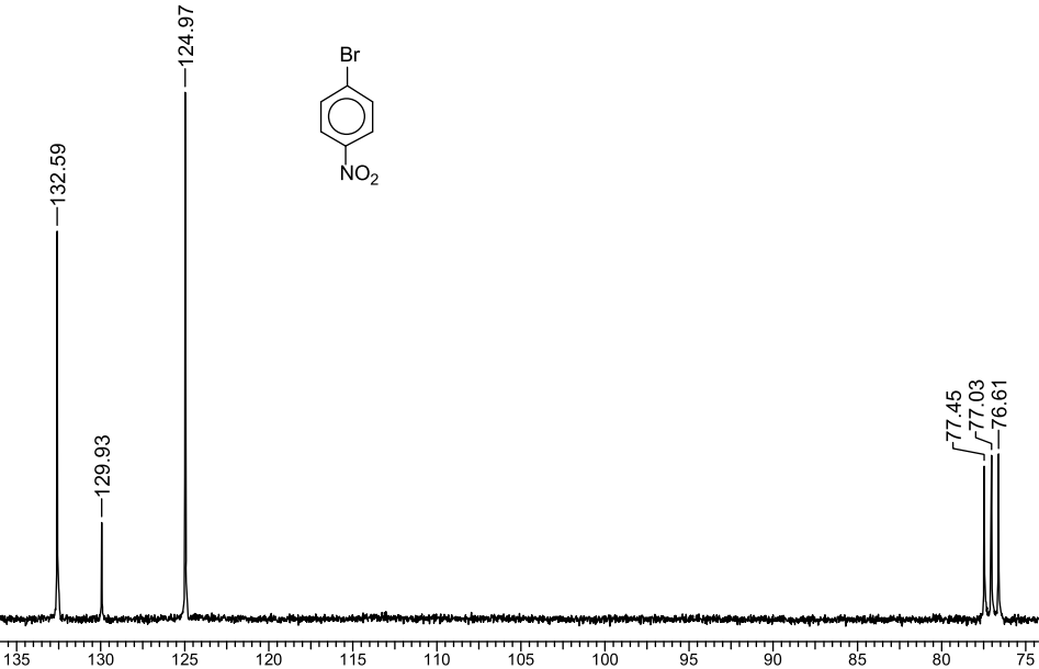
Б7.1.1. Спектры ЯМР ^1\text{H} и ^{13}\text{C} 1-бром-4-нитробензола
