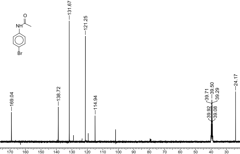
Б7.2.5. Спектры ЯМР ^1\text{H} и ^{13}\text{C} N-(4-бромфенил)ацетамида
