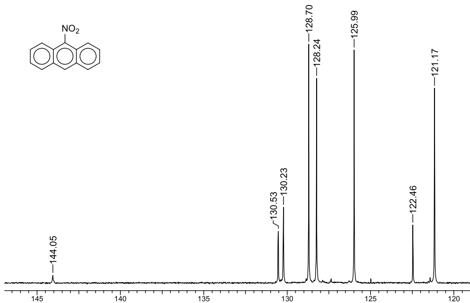
Б7.1.8. Спектры ЯМР ^1\text{H} и ^{13}\text{C} 9-нитроантрацена
