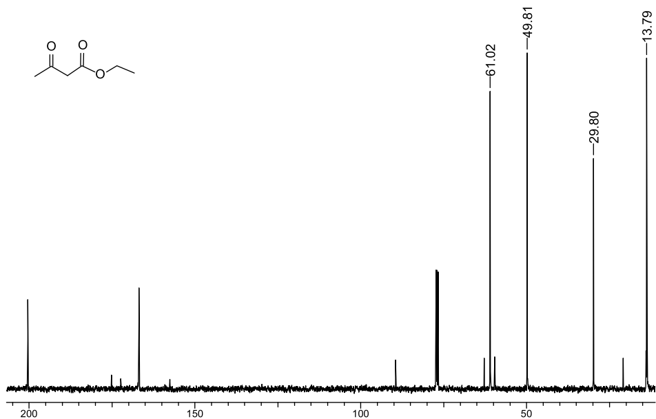
В5.3.3. Спектры ЯМР 1 H и 13 C этил-3-оксобутаноата
