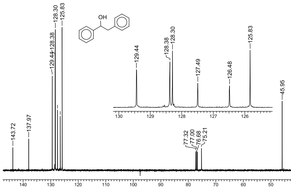
Б6.4. Спектры ЯМР 1 H и 13 C 1,2-дифенилэтанола
