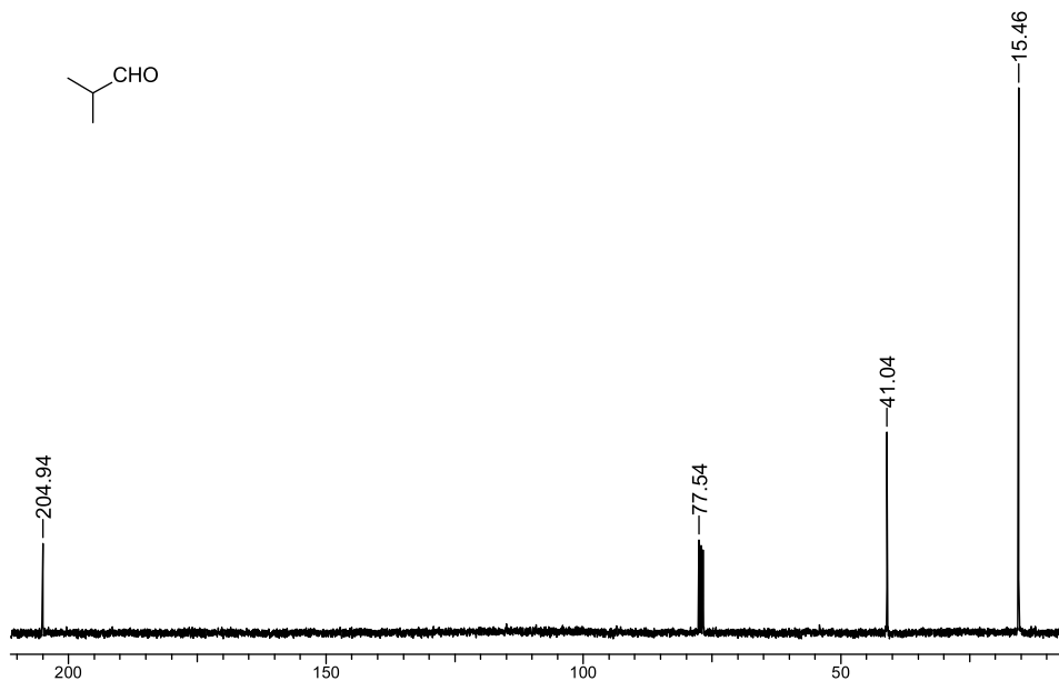
Б4.1.2. Спектры ЯМР ^1\text{H} и ^{13}\text{C} 2-метилпропаналь
