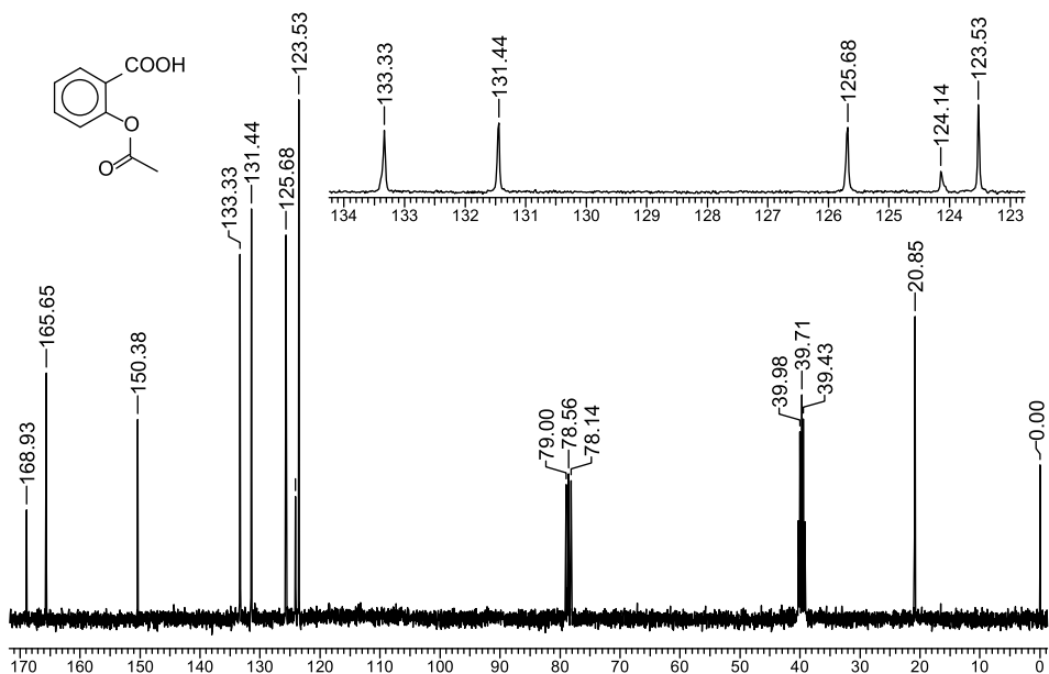
Б1.1.8. Спектры ЯМР ^1\text{H} и ^{13}\text{C} 2-(ацетилокси)бензойной кислоты
