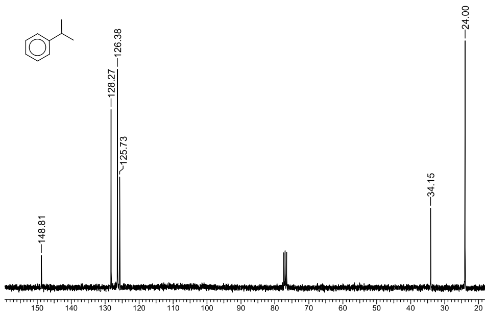
Б7.8.1. Спектры ЯМР 1 H и 13 C изопропилбензола
