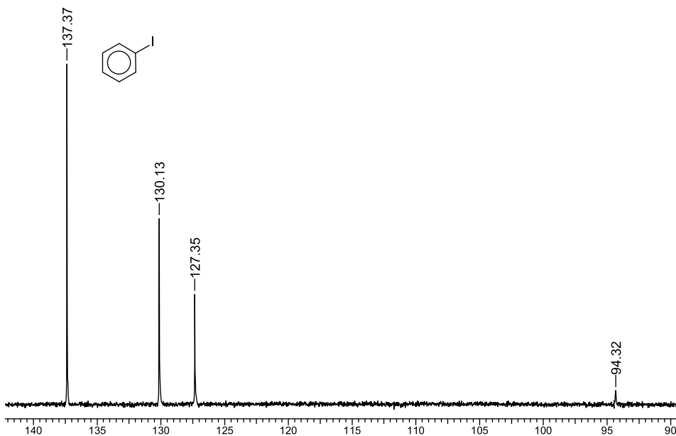
Б10.1. Спектры ЯМР 1 H и 13 C иодбензола
