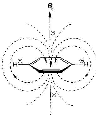
Рис. 54. Диамагнитный кольцевой ток в бензоле
