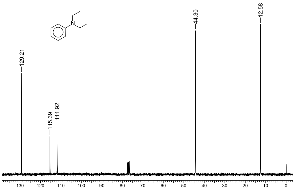
Б3.4.2. Спектры ЯМР 1 H и 13 C N,N-диэтиланилина
