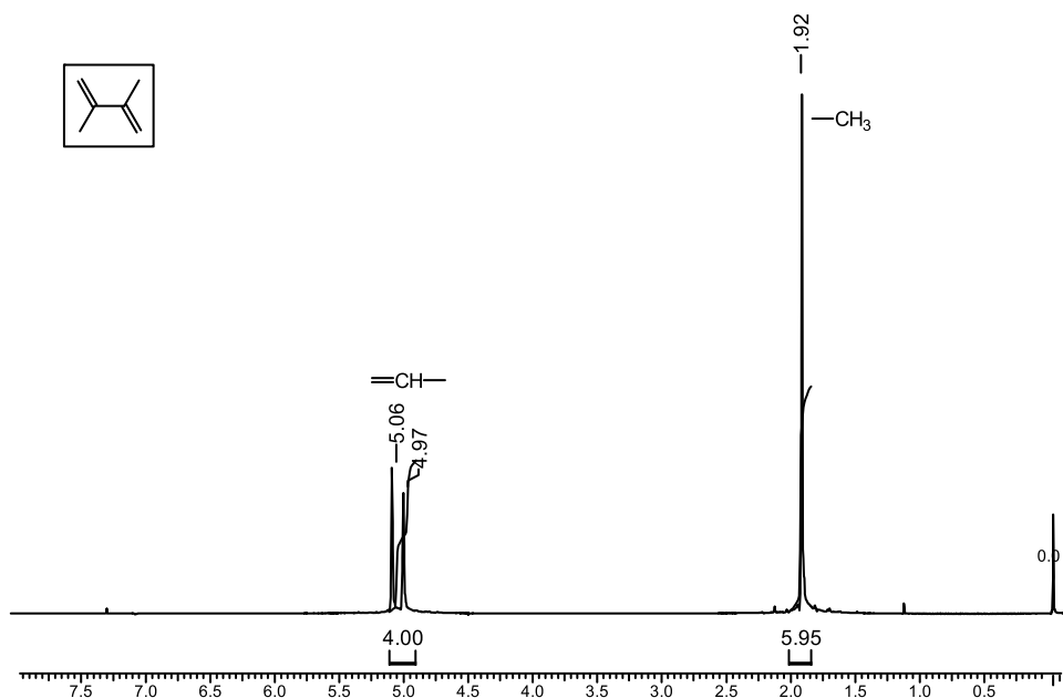
Рис. 51. Спектр ЯМР ^1H 2,3-диметилбутадиена-1,3
