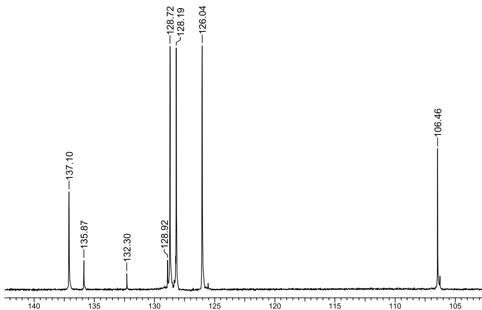
Б2.1.6. Спектры ЯМР 1 H и 13 C (2-бромэтил)бензола
