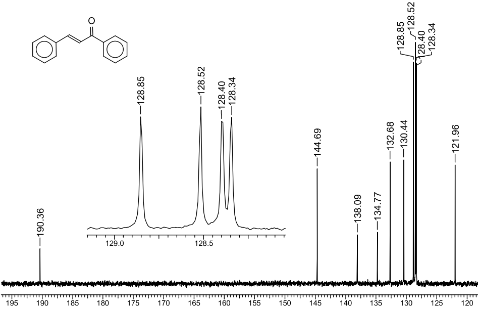
Б4.3.4. Спектры ЯМР 1 H и 13 C (2E)-1,3-дифенил-2-пропен-1-она
