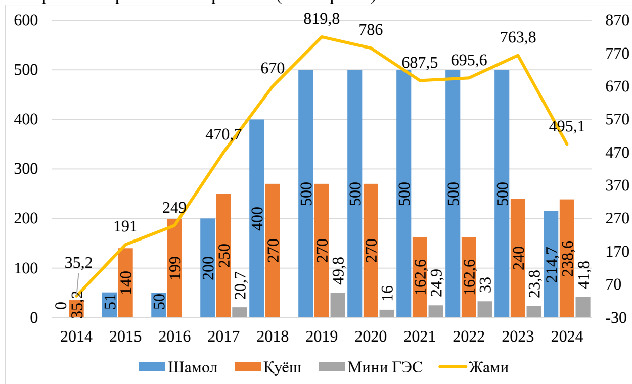
9.3.2-расм. Россияда тикланадиган энергия манбаларини ўзлаштириш қувватларини ишга туширишнинг мақсадли кўрсаткичлари, МВт
