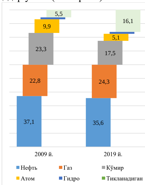
8.4.2-расм. Германияда бирламчи энергия истеъмоли таркибининг ўзгариши, % 228
