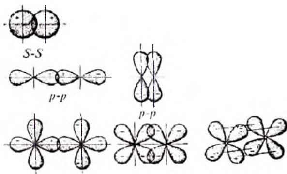
15-rasm. \sigma -, \pi - va \Delta - bog'larining hosil bo'lishida elektron bulutlarning qoplanish sxemasi.
