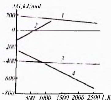
2-rasm. Kimyoviy reaksiyalarning izobar izotermik potensialining qiymatining haroratga bog'liqligi:
