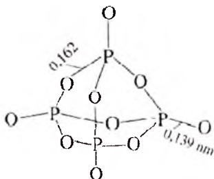
46-rasm. Fosfor (V) oksid molekulasi tuzilishi.
