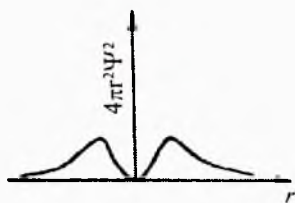
10-rasm. 2p- elektronlarning radial taqsimlanish ehtimoligini ko'rsatuvchi egri chiziqlar.
