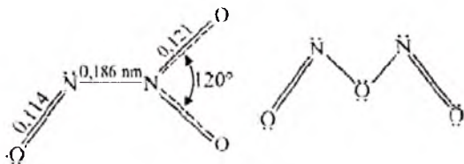
43-rasm. Azot (III) oksidi molekulasining tuzilishi.
