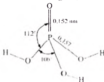
47-rasm. Ortofosfat kislota molekulasi tuzilishi.
