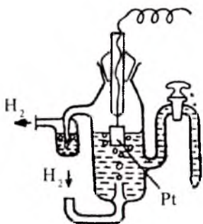
31-rasm. Vodorod elektrodining ko'rinishi.
