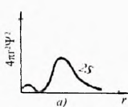
8-rasm. 2s- va 3s- elektronlarning radial taqsimlanish grafigi.
