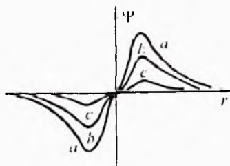
9-rasm. 2p- elektronlarning to'liq funksiyasi grafigi.
