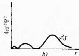
8-rasm. 2s- va 3s- elektronlarning radial taqsimlanish grafigi.
