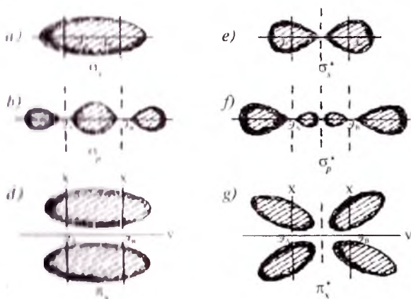
22-rasm. Ikki atomli molekularlarning molekular orbitallari: a, b, d — bog'lovchi \sigma_p — molekular orbitallar; e, f, g — bo'shashtiruvchi \sigma_p^* — molekular orbitallar; d — bog'lovchi \pi_p va e — bo'shashtiruvchi \pi_p^* — orbitallar.
