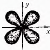
12-rasm. 3d- elektronlar bulutining fazoviy shakli.
