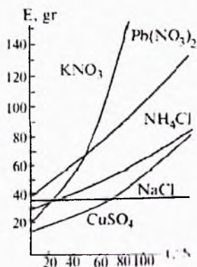
3-rasm. Eruvchanlik egri chiziqlari.
