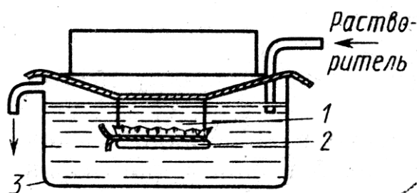
Схема диализатора.
