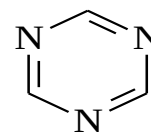
triazin
