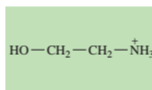
Этаноламин
