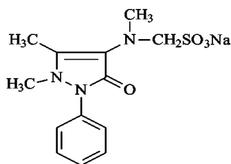
Анальгин
