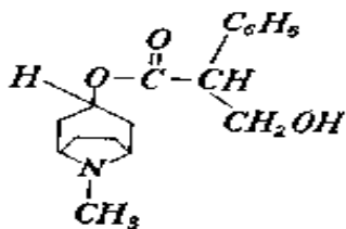
Атропин
