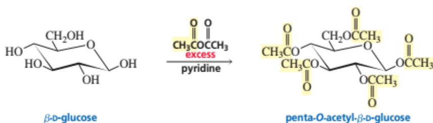
D-глюкопираноза 1,2,3,4,6-Пента-О-ацетитил-D-глюкопираноза (пентаацетилглюкоза)
