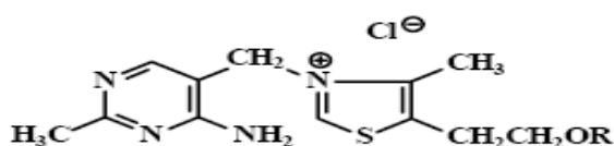
Тиаминмонофосфат
