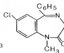
Диазепам
