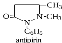
antipirin
