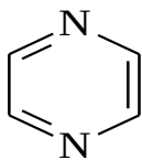
pirazin
