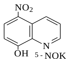
8-Гидрокси-5- нитро- хинолин (5-НОК)
