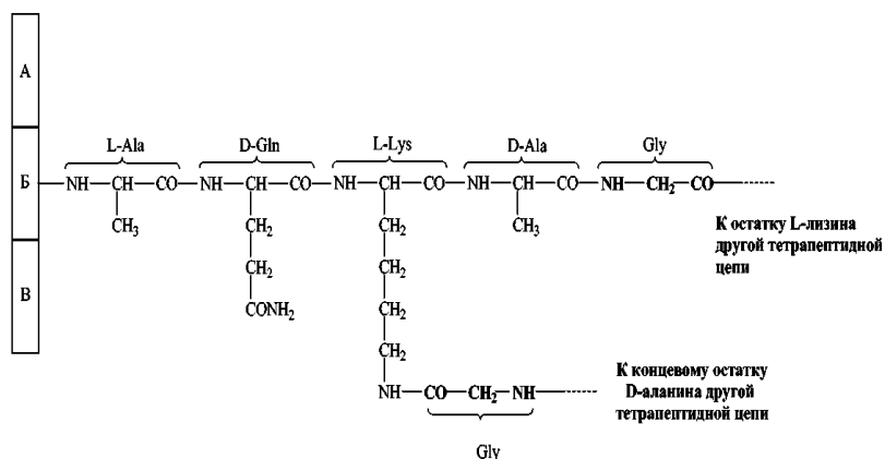
Строение тетрапептидной цепи муреина.
