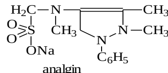
analgin
