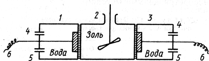
Схема электродиализатора.
