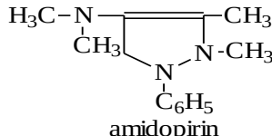
amidopirin
