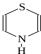
tiazin
