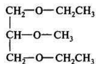
2-метокси-1,3-диэтоксипропан (a)
