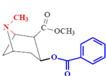
Кокаин
