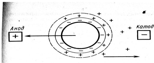
Схема движения коллоидной частицы в электрическом поле.
