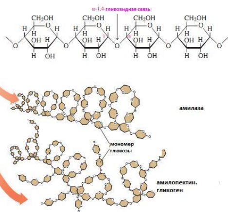
Разветвленная макромолекула амилопектина.
