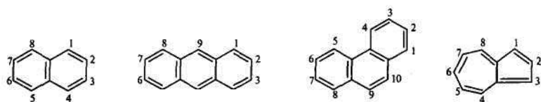
нафталин антрацен фенантрен азулен
