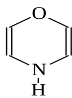
oksazin
