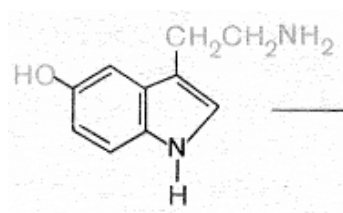
Серотонин (5-гидрокситриптамин)
