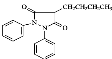
Бутадион
