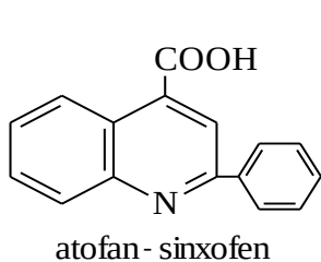
Атофан
