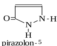
pirazonon -5
