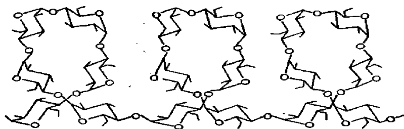
Спиралевидная цепь амилозы.
