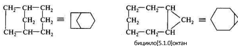
бицикло[3.2.1]октан
