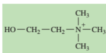
холин
