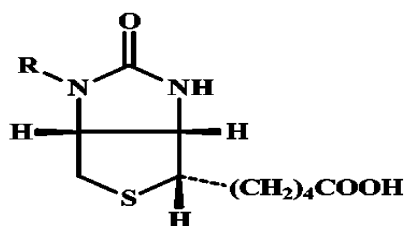
Витамин Н (биотин) N 5 -Карбоксибиотин
