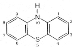
Фенотиазин
