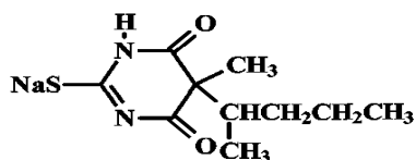
Тиопентал натрий
