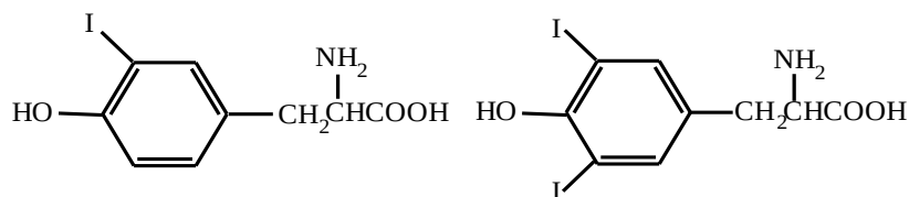
3-Йодтирозин
