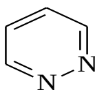
piridazin
