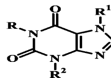
Кофеин R=R^1=R^2=CH_3 Теобромин R=H; R^1=R^2=CH_3 Теofilлин R=R^2=CH_3; R^1=H
