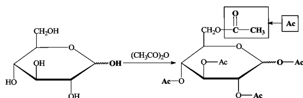
D-глюкопираноза 1,2,3,4,6-Пента-О-ацетитил-D-глюкопираноза (пентаацетилглюкоза)
