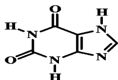
Ксантин
