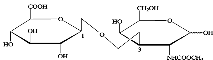
D-глюкоурановая кислота N-ацетил-D-галактозамин N-ацетилхондрозин
