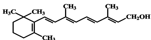
Витамин А
