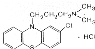
Аминазин
