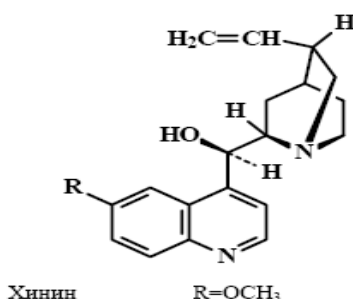
Хинин
